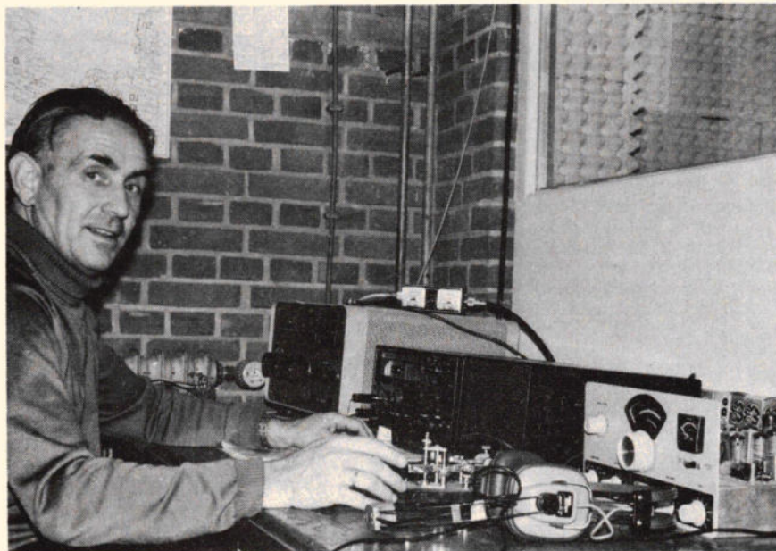
De VERON-verenigingszender PAoAA in de toren van de Sikkens lakfabrieken te Sassenheim. Van hieruit worden wekelijks uitzendingen voor de Nederlandse amateur verricht, o.a. morsecursussen. Achter de apparaten: de eerste operateur van dit station, OM van Weerlee, PaoYZ. (Helaas alleen maar gekochte spullen en niets meer van dat zelfgemaakte; als enige concessie aan het amateurchap is van één apparaat de kast verwijderd). De VERON heeft 40 landelijke afdelingen, in veel gevallen met afdelingszender.
